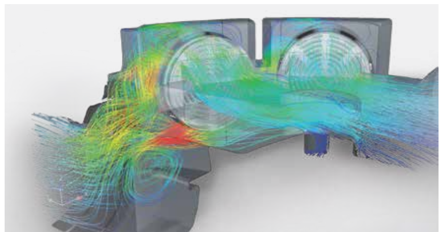
Fluid-dynamic evaluation
